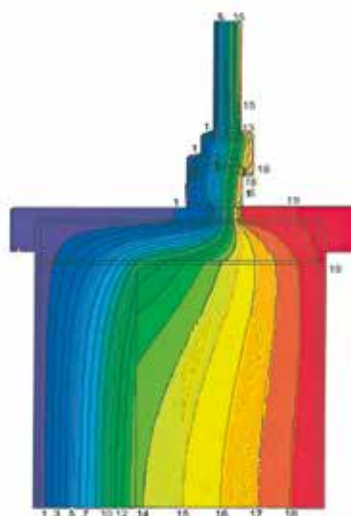
Campo temperature densità flusso termico
