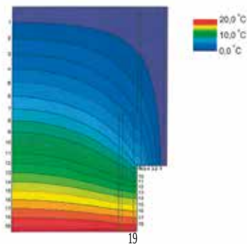
Campo temperature densità flusso termico
