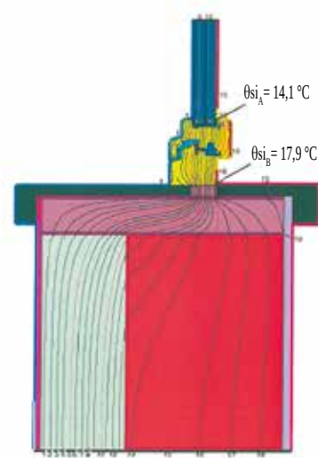
Temperature nei punti critici
