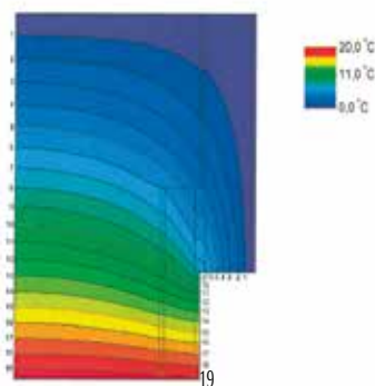
Campo temperature densità flusso termico
