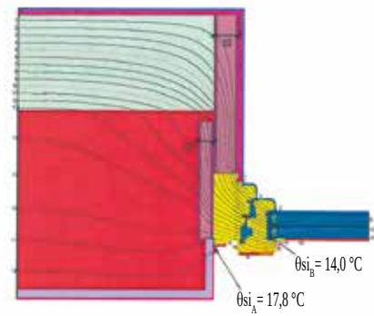
Temperature nei punti critici
